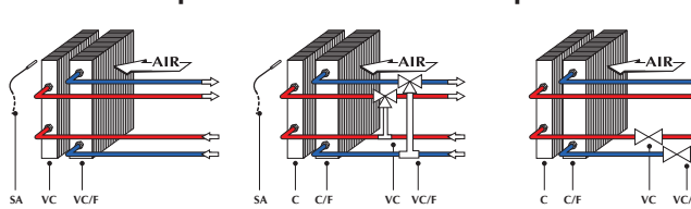
Impianto 4 tubi senza sonda acqua
