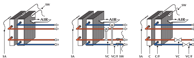
Instalación de 4 tubos con sonda agua
