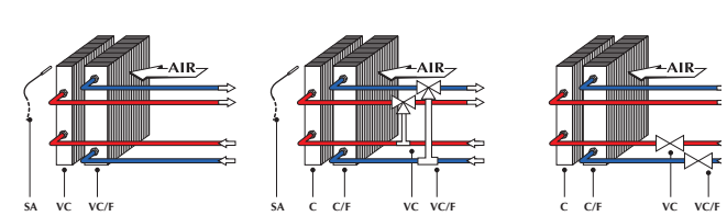
Instalación de 4 tubos sin sonda agua
