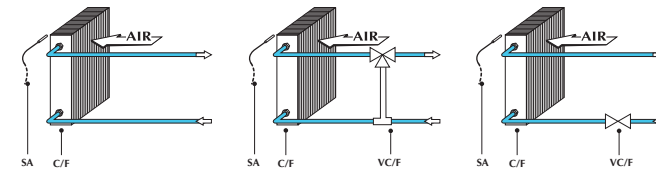
Instalación de 4 tubos sin sonda agua
